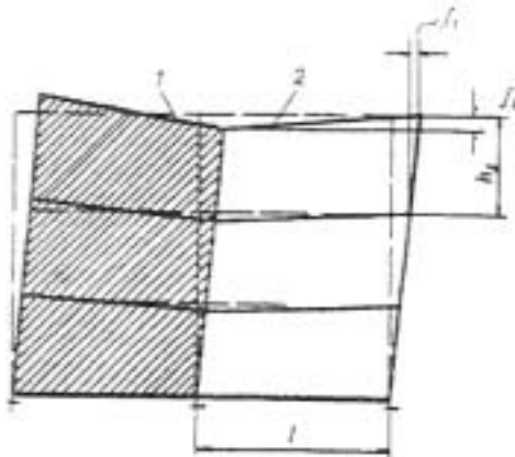
Черт. 6. Схема перекоса этажных ячеек 2, примыкающих к диафрагмам жесткости I в зданиях со связевым каркасом (пунктиром показана исходная схема каркаса до приложения нагрузки)
